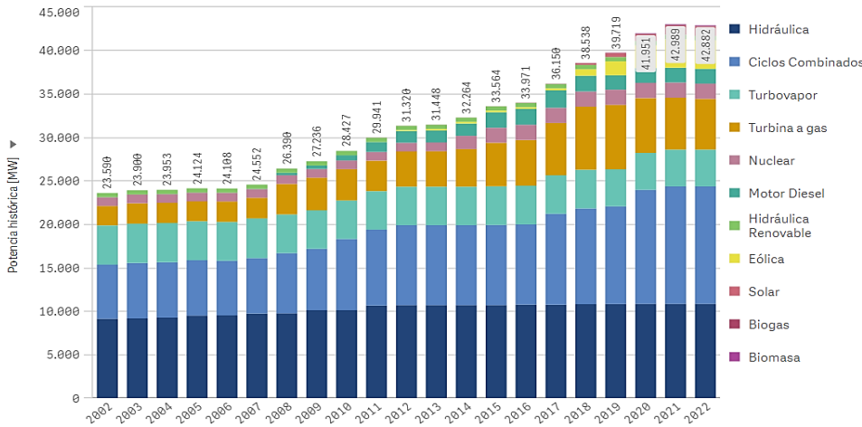
Ilustración 1 - Proyecciones de potencia instalada - Período 2002 / 2022 (Fuente: CAMMESA)
